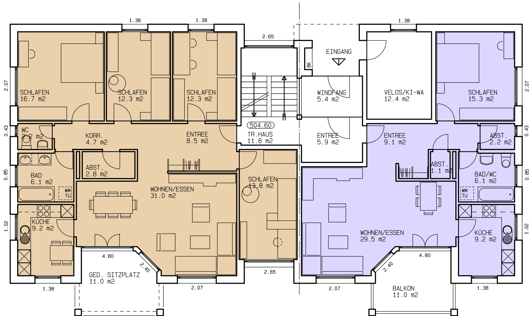
② Typ 3 5 1/2 ZI-WG (ROLLSTUHLGÄNGIG) Nettonutzflächen=119.6 m 2 (exkl. ged. Sitzplatz)
