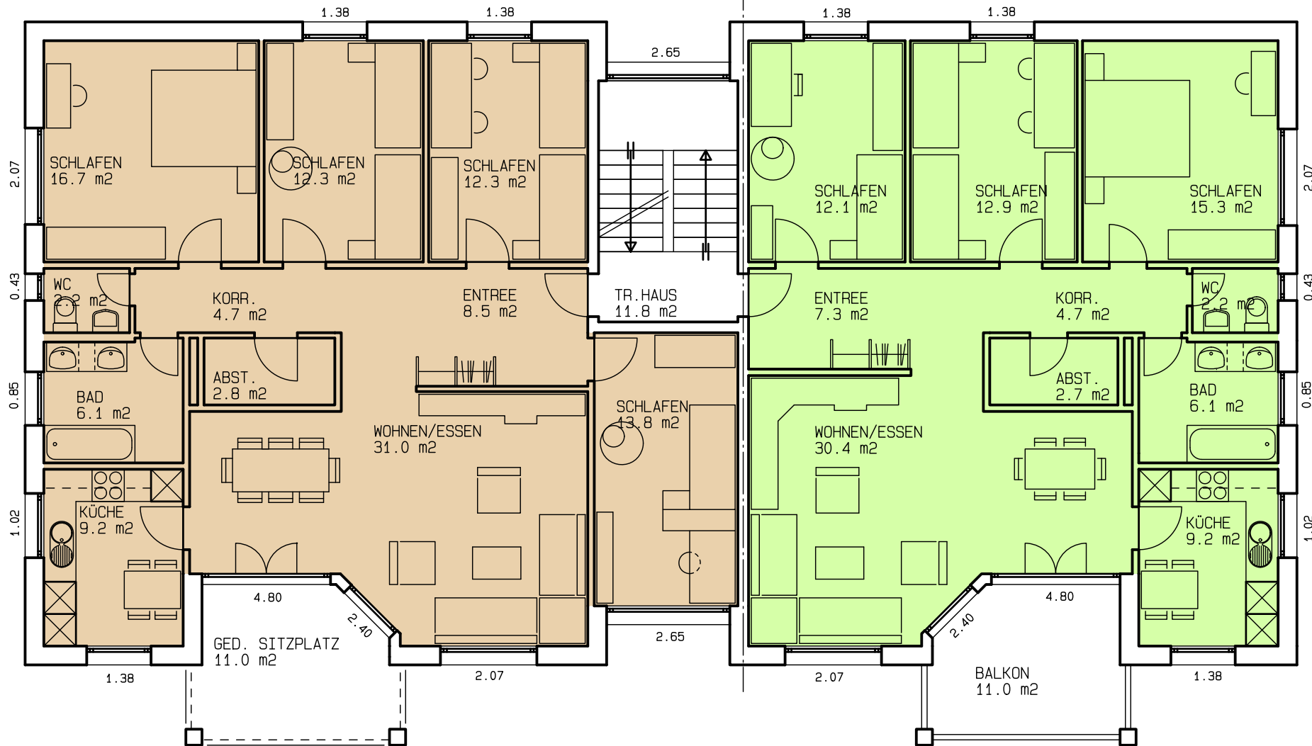
② Typ 3 5 1/2 ZI-WG Nettonutzflächen=119.6 m 2 (exkl. ged. Sitzplatz)
